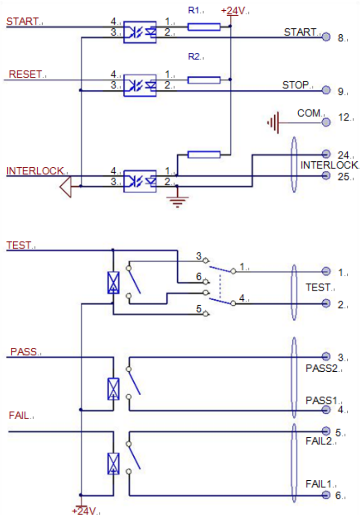
图 9-2 仪器 Handler 接口内部电路结构
