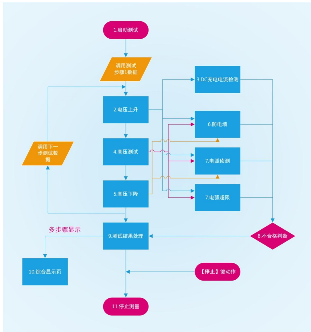
图 5-2 测试流程图
